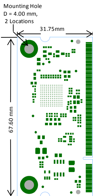
Module Dimensions
